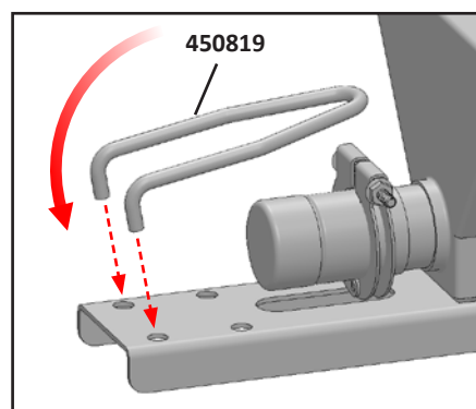
Ensamble el gancho paso 1
