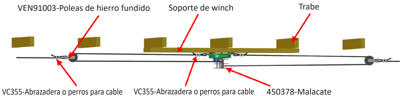
FIGURA 4A (Vista detallada de la elevación doble trasera)
