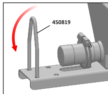
Ensamble el gancho paso 2
